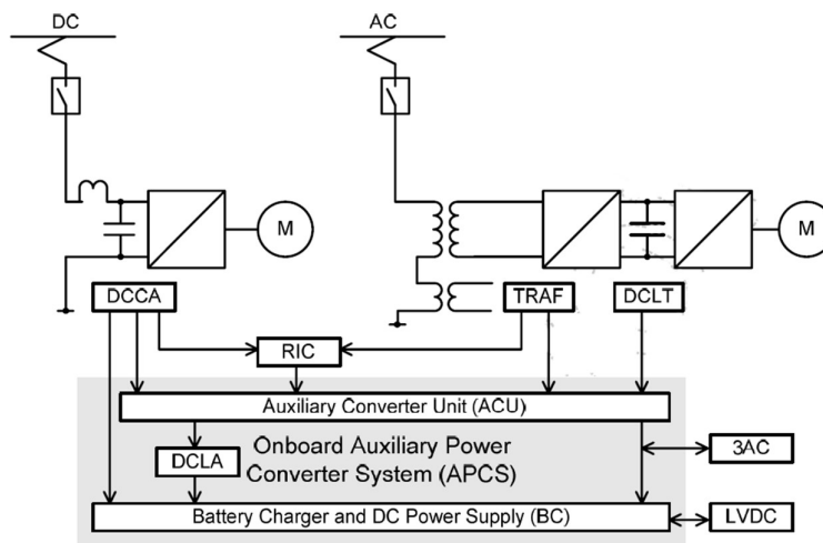
Rysunek 18 Typowy interfejs przetwornicy statycznej w pociągu.
