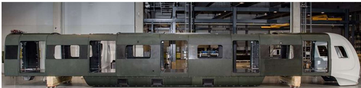
Rysunek 10 Widok nadwozia pojazdu metra wykonanego z kompozytu CFRP [7]
